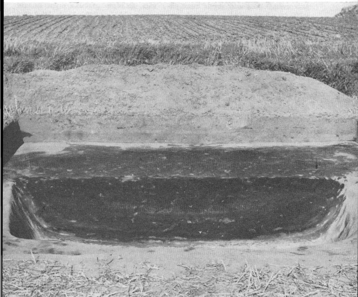
Snitt genom ett av grophusen på Hagestad nr 19. Det från början djupt nedgrävda golvet har etappvis höjts, sannolikt av hygieniska skäl, och man har varje gång täckt golvytan med halm e. d.
