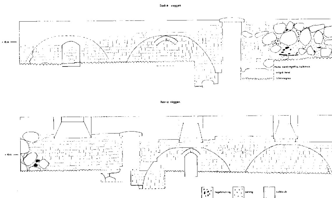
Gråbrödraklostret i Ystad. Uppmätningsskiztning av norra längans fasader mot söder och norr, rum B och C.
