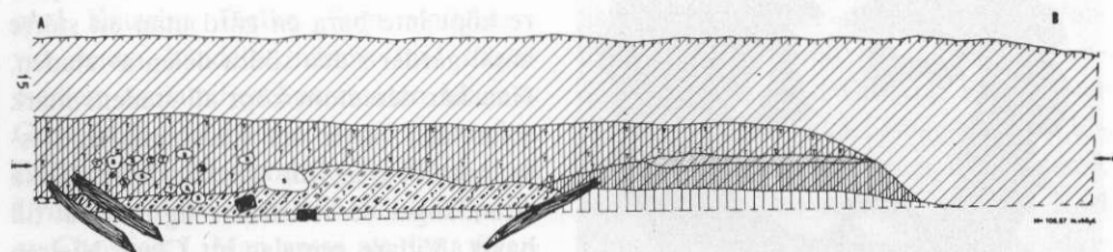
Fig 4. Profil genom vällen. Strandskoningarna av ekpålar har pressats utåt. Uppmätningar av förf.
