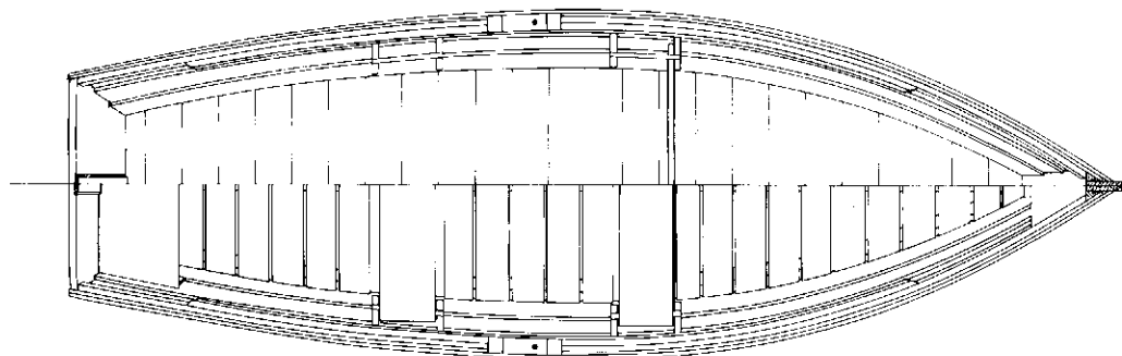
Uppmättningsritning. Flateka byggd av Edgar Sundén i Kristianopol under våren 1980.
