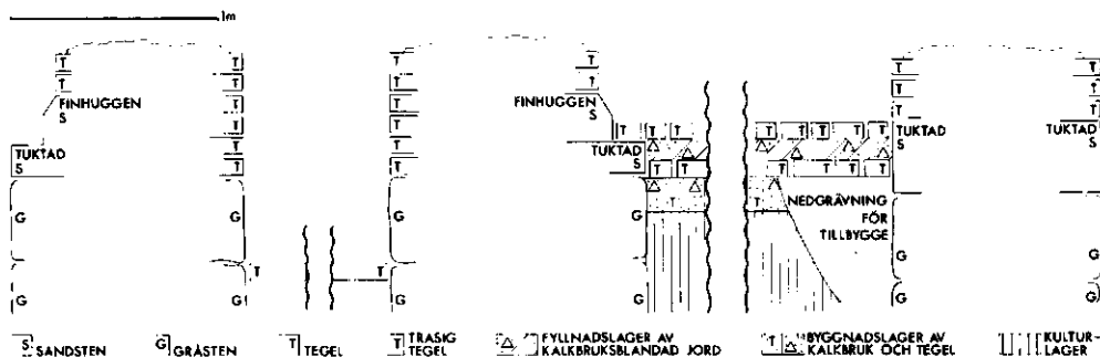
Fig. 1. Schematiserad sektion mot väster, genom huvudbyggnadens södra och norra samt tillbyggnadens norra mur. Sektionen är en sammanställning av ritningar från 1955 och 1979 års undersökningar.
