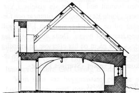
Fig. 2. Sektion genom Ostkällaren, kv. Färgaren, Varberg. Uppmätt av B. Wetter 1964.
