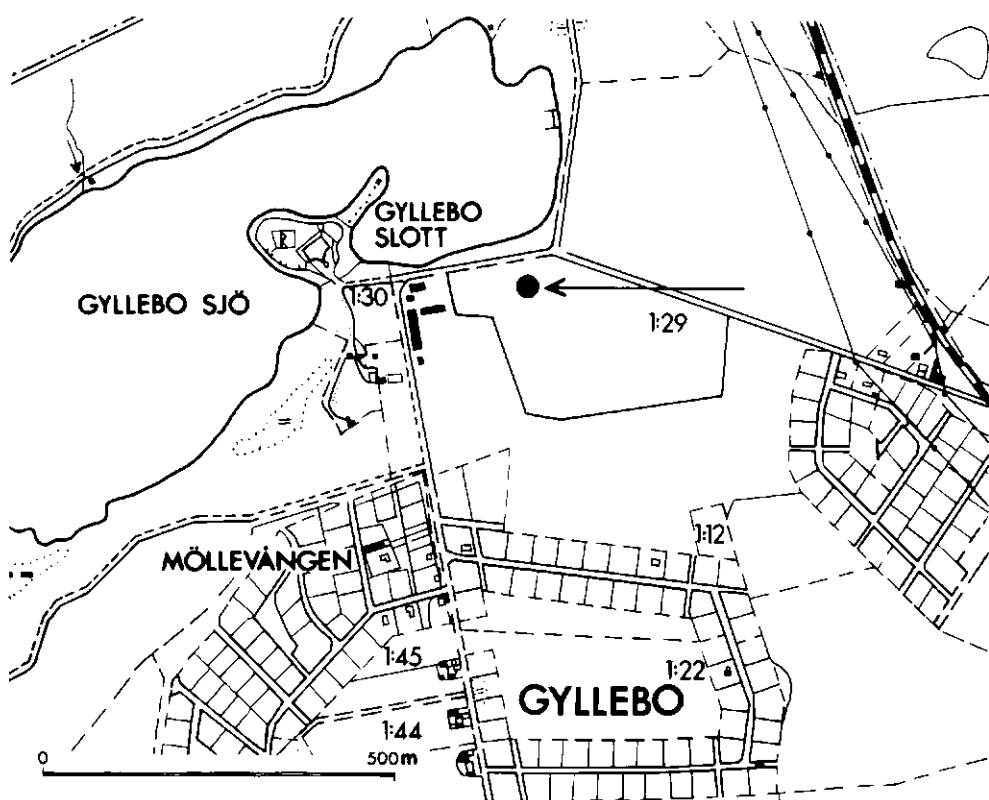
Fig. 1. Kartskiss med fyndplats för solidus markerad.
