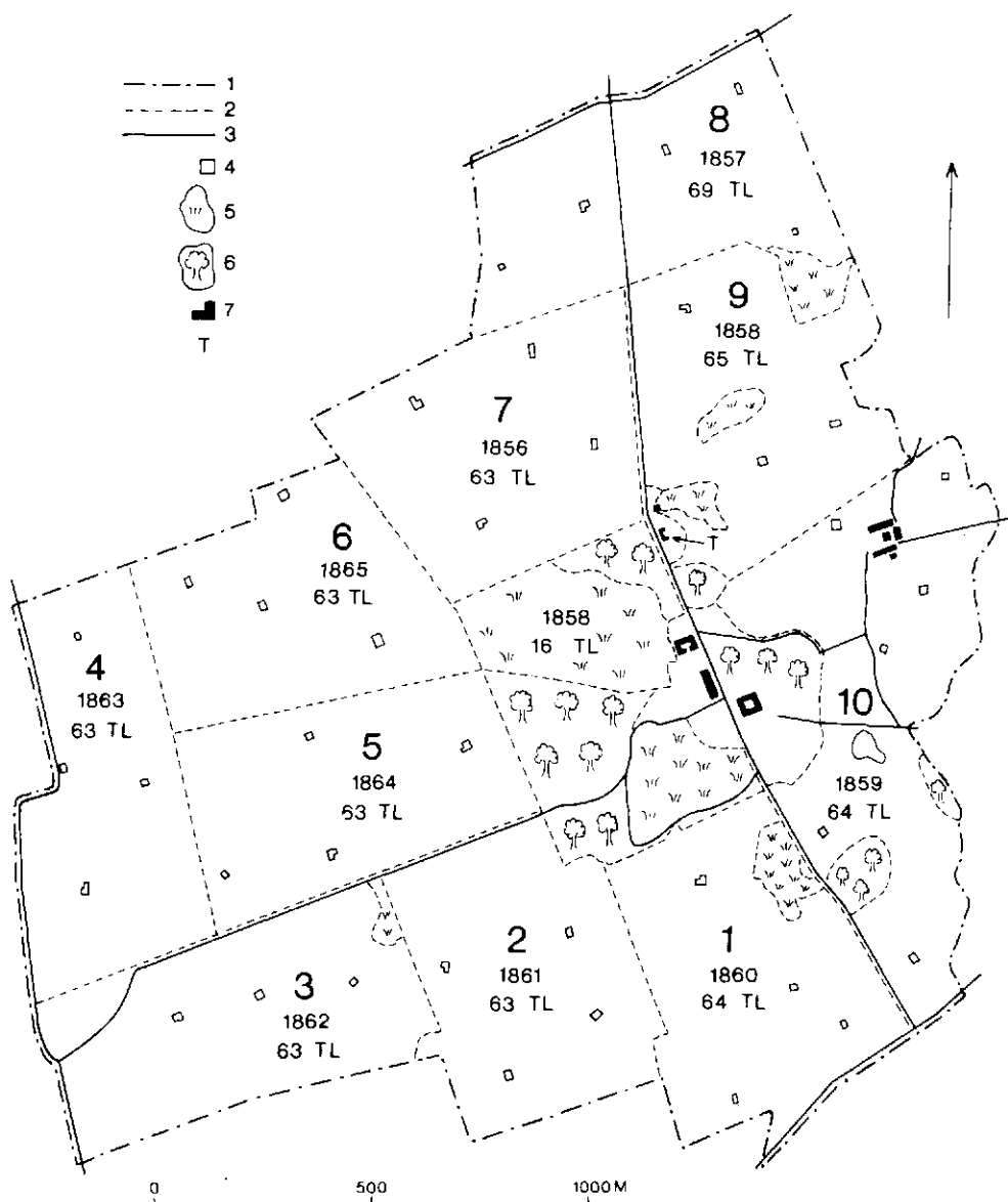
Fig. 7. Täckdikning på Charlottenlunds gods 1856–66. 1=yttre gräns för mark under godsets drift, 2=vånga-gräns, 3=vägar, 4=märgelgravar, 5=äng, 6=skog, 7=byggnad och T=tegelbruk. Källa: Kartor förvarade på godset.
