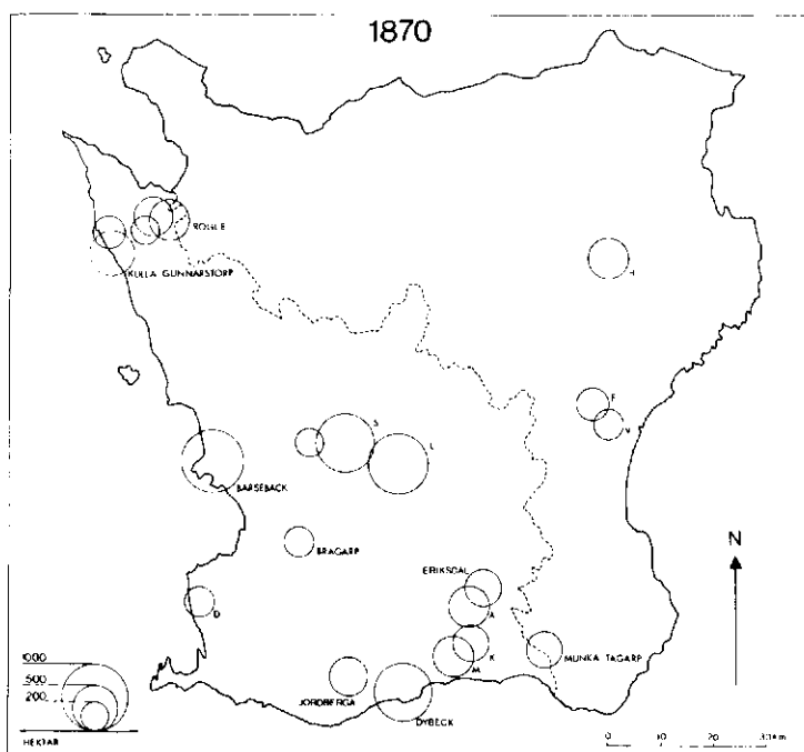
Fig. 3-6. Dikningsarbeten i Skåne utförda av lantbruksingenjör Åkerman och hans medarbetare 1865-79. Varje karta redovisar de enheter som t.o.m. respektive år sammanlagt dikat mer än 200 hektar. Källa: Lantbruksingenjörens årsberättelser.
