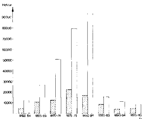
Fig. 2. Grunddikning i Skåne 1860–99. Mörk stapel=Kristianstads län, ljus stapel=Malmöhus län. Källa: Bidrag till Sveriges Officiella Statistik, N) Jordbruk och Boskapsskötsel.
