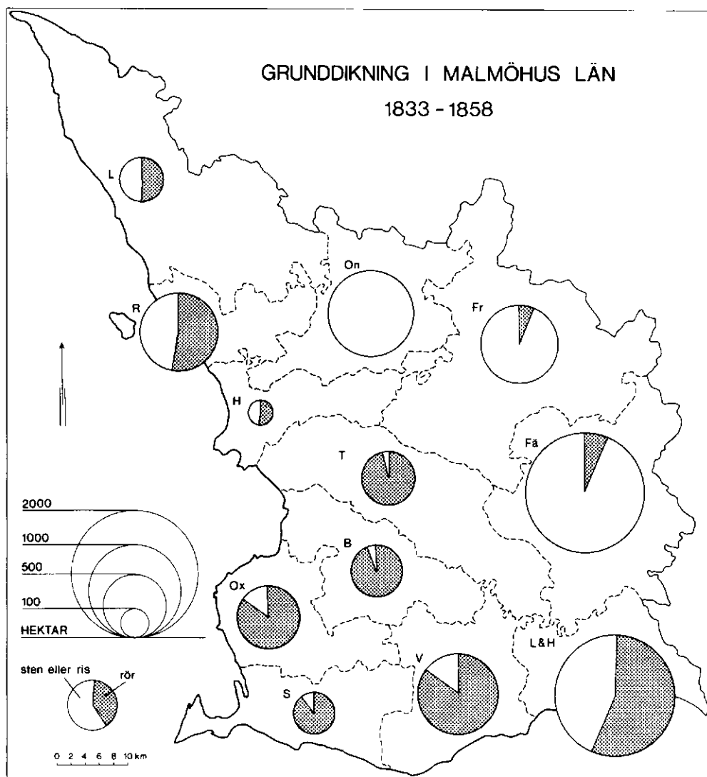
Fig. 1. Grunddikning i Malmöhus län 1833-58. Källa: Tidning för Landthushållning 1858.
