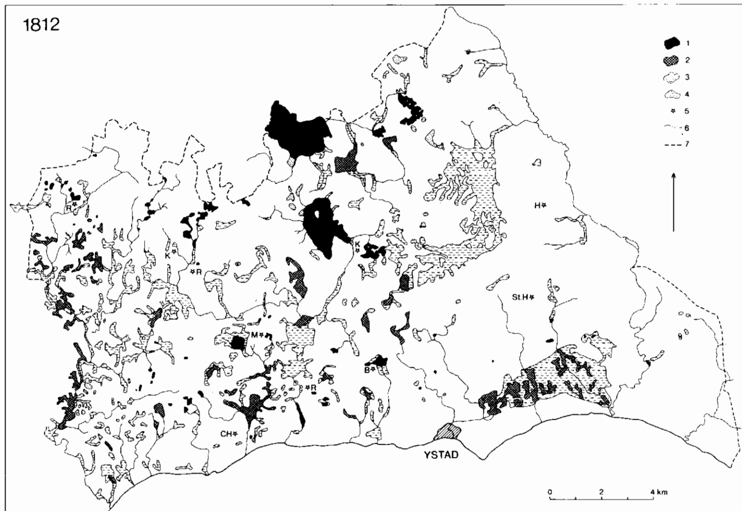
Fig. 8. Våtmarker i Ljunits och Herrestads häraders år 1812. 1=öppet vatten, 2=sankt kärr, 3=kärr/mosse, 4=öppen alskog av skottskogskaraktär på fuktäng, 5=huvudbyggnad på gods, 6=vattendrag och 7=områdesgräns som inte sammanfaller med vattendrag. Renritning efter Skånska Rekognosceringskartan.
