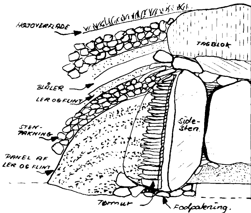
Fig. 4. Schematisk snitt gennem høgens fyllning bakom kammarens sidosten. Svend Hansen 1986.
