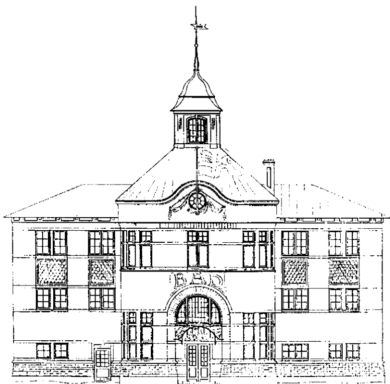
Karlskrona varmbadhus. Nybyggnadsritning 1903, västra fasaden.
