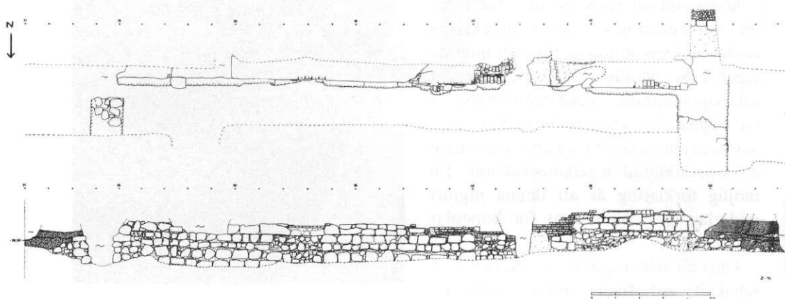
Fig. 5. Plan- och sektionsritning över långhusets grund- och dagermur. Sektionen är sedd från norr. Renritning: P. Carelli.
