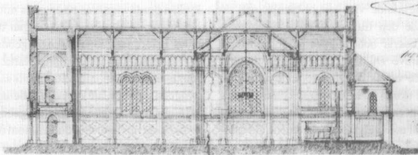
SNIT m. E.F.
