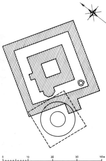
Fig. 3. Plan av Kärnan och dess skyddsmur. I det södra hörnet innanför skyddsmuren finns en brunn. Cirkelarna markerar det äldre rundtornet. Den streckade linjen utanför dem anger en sekundär förstärkning (se sid. 11). Ritning av Ulla Benander.
