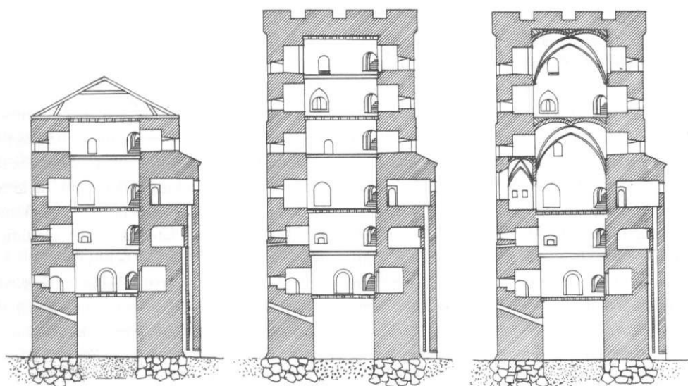
Fig. 4. Rekonstruerade höjdsektioner av Kärnan, visande tornet efter det första byggnadsskedet resp. efter fullbordandet och förändringen av de översta våningarna. Det ofullbordade tornet var antagligen försett med en provisorisk taktäckning. Murkrönet på det färdiga tornet är fritt rekonstruerat. Ritningar av Annika Cronsioe efter anvisn. av förf.
