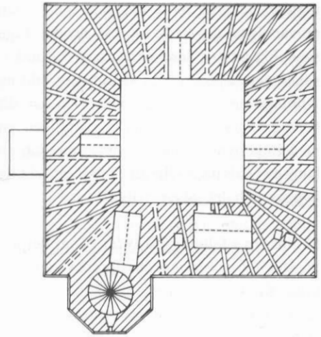
Fig. 8. Plan av Kärnan på tjugo meters höjd, visande hur de stora bomhålen går igenom eller har gått igenom hela murverket (streckade bomhål är delvis igenfyllda). Ritning av Mårtensson, 1934.
