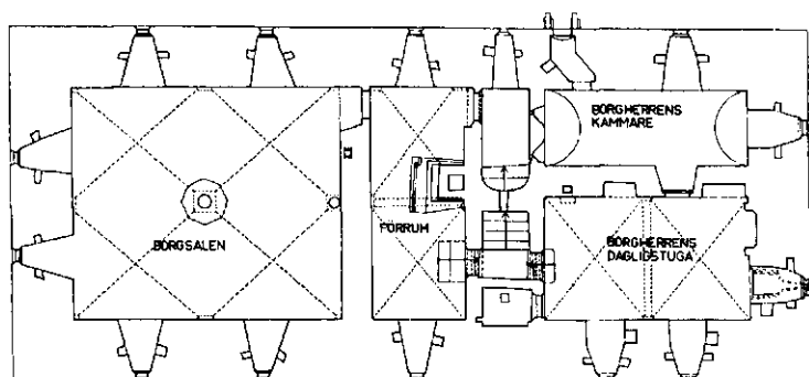
Plan over første etage. Efter opmåling af Sten Anjou 1925.
