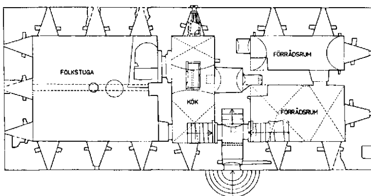
Plan over kælderens. Bemærk indgangsdøren til højre på planen. Efter opmåling af Sten Anjou 1925.
