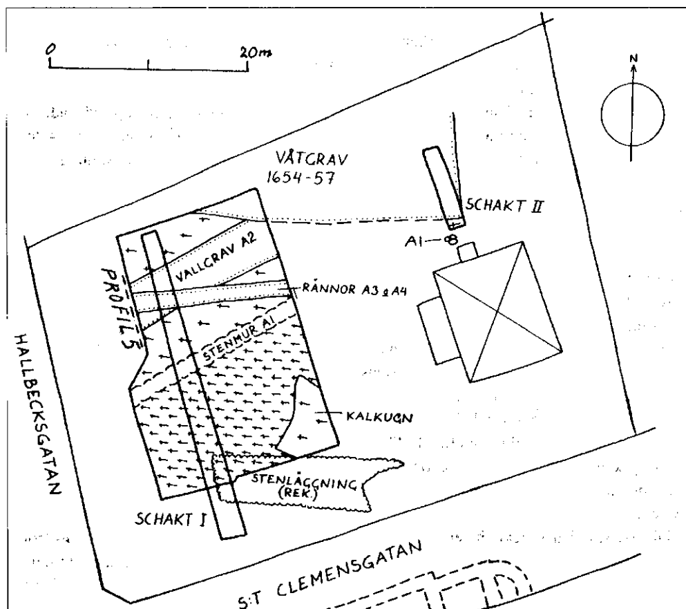
Fig. 2. Situationsplan med provschakt från förundersökningen och 1987 års undersökningsyta, där vallgravsprofilen 5 är streckad liksom S:t Clemens kyrka nedtill på bilden. (Anglert 1996, fig 3.)
