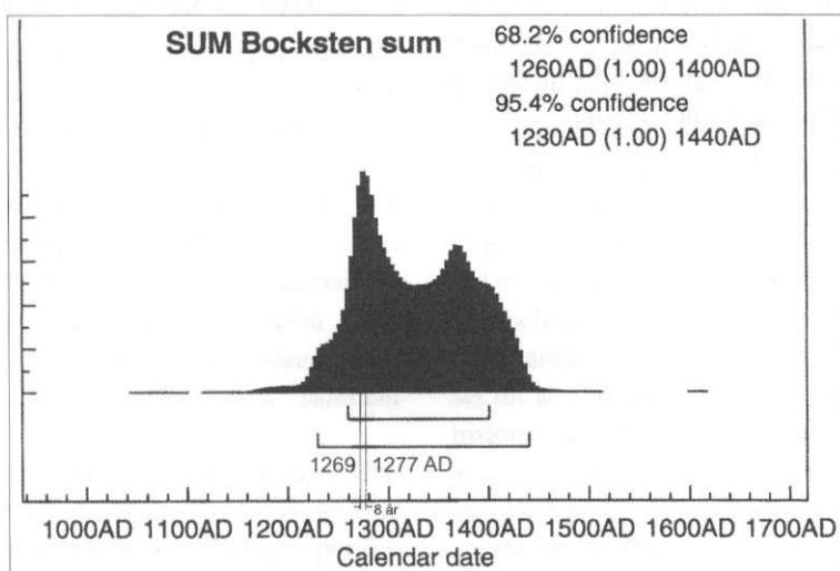
9. Diagrammet visar sannolikhetsfördelningen av daterade prover (17) från Bockstensfyndet, som utförts fram till 1997. Den större kurvan till vänster anger den verkliga dateringen, medan kurvan till höger är en skenbar datering av Bockstensfyndet. Årtalen AD 1269 och AD 1277 är införda som referensårtal för att lättare kunna bedöma dateringen på den horisontella tidsaxeln. Det mest sannolika dateringsintervallet har hamnat på perioden 1250–1295 AD. Dateringskurvan för detta prov är hämtad från boken Bockstensmannen och hans dräkt, 1997, sid 136.
