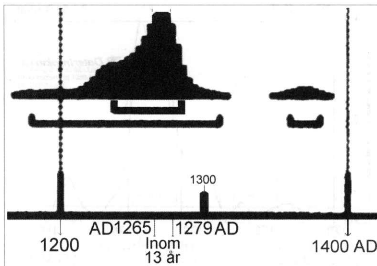
7. Diagrammet återger dateringen av prov från kjorteln ullfibrer, enligt lab nr Ua-11095. Dateringen har hamnat på 740 \pm 45 BP, vilket motsvar års- intervallet 1250–1290. Maxvärdet eller väntevärdet har hamnat på ca 1265–1279 AD med en spridning inom ca 13 år. Även här framträder en mindre dateringspuckel, som till höger, är en skenbar effekt av kalibreringskurvens olinjäritet under 1300-talet. Källa: Bockstensmannen och hans dräkt, 1997, sidorna 125–136.
