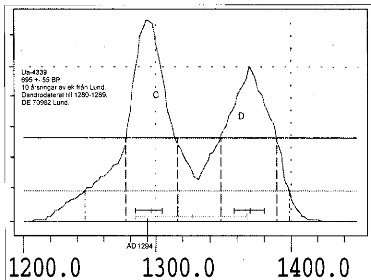
4. Diagrammet visar C14-datering av tio årsringar från en ek, som med säkerhet är dendrokronologiskt daterad till årsintervallet 1280–1289 AD (DE 70982 Lund). Dateringen visar två sigma (C och D). Den vänstra kurvan (C), som har maxvärdet ca AD 1294, visar i det här fallet att C14-metoden ger något för låg ålder (ca 10 år) i jämförelse med den säkrare dendrokronologiska åldersbestämningen. Den högra kurvan (D) visar således en falsk eller skenbar datering. Dateringen utförd av Tandemlaboratoriet i Uppsala 1994 med lab nr Ua-4339, 695 \pm 55 BP.
