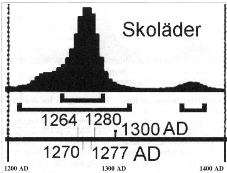
5. Diagrammet visar C14-dateringen av Bockstensmannens skoläder, enligt prov Ua-11091. Kurvens maxvärde eller väntevärde har hamnat på årsintervallet AD 1270–1277, med en spridning från ca 1260–95. Den betydligt lägre puckeln t h har hamnat på andra hälften av 1300-talet och utgör en skenbar datering p.g.a. kalibreringskurvens ojämnhet.
