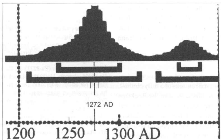
8. Diagrammets vänstra kurva återger dateringen av ullfibrer från Bockstensmannens struthätta, enligt lab nr Ua-11097, 715 \pm 50 BP. Väntevärdet har hamnat på ca 1265–1280 AD, som överensstämmer med övriga dateringar. Den mindre kurvan till höger är således en falsk datering pga kalibreringskurvens ojämnheter. Källa: se diagram 7.
