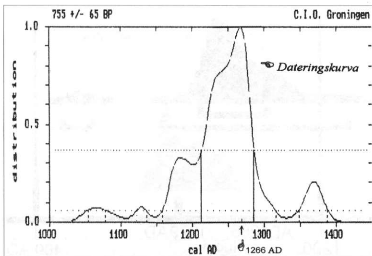
6. Diagrammet visar resultatet av C14-dateringen av Bockstensmannens klädeklädd (Ua-2439). Detta dateringsprov har förbehandlats i tre steg för att eliminera eventuella föroreningar, som kan påverka dateringen. Dateringskurvens max- eller väntevärde har hamnat på AD ca 1266. Vid jämförelse med diagram 1 är tidsskillnaden (1330–1266) ca 65 år, som tidsförskjutningen framåt utgör. Denna tidsförskjutning har uppstått även på de senaste dateringarna, som exempelvis Ua-32333 (ull kjortel), 32334 (ull fotlapp) och 32337 (lårben), dock i mindre omfattning (20–40 år). Källa: Tandemlaboratoriet i Uppsala 1992 och 2006.
