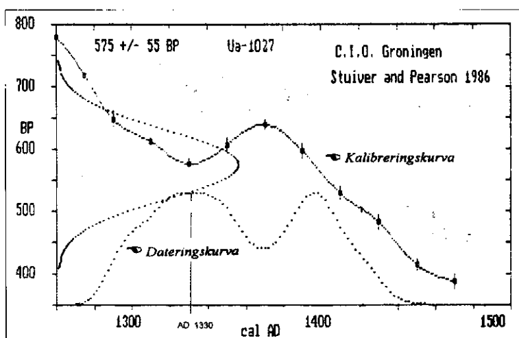
1. Diagrammet visar resultatet av en av de första C14-dateringarna av Bockstensmannens klädeklädd från 1988. Lab nr Ua-1027, som utgör textilprov B. Kemisk förbehandling, enligt alternativ a. Ursprunglig vikt = 8,00 mg. 1. behandling i 1 % HCl, 80°C, 3 timmar. 2. tvättning i destillerat vatten. 3. torkning. Vikt efter preparation = 7,46 mg. Den procentuella viktminskningen = 6,75 %. Preparationsdatum 1988-11-14. En markeringslinje vid året AD 1330 är inlagd i syfte att användas vid jämförelse med diagram 6. Källa: Tandemlaboratoriet i Uppsala, Ua-1027.
